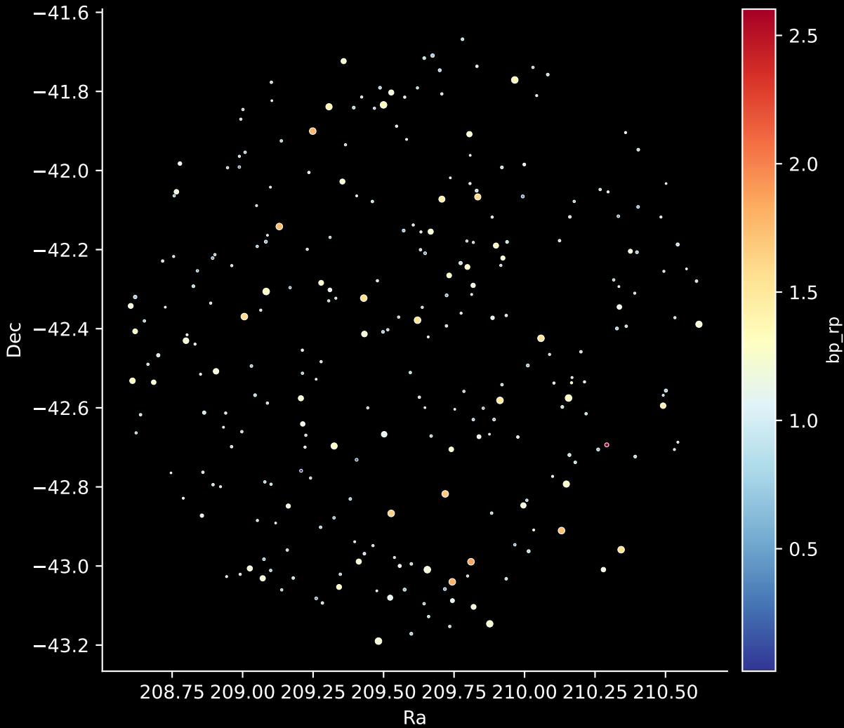
GALAH DR4 Field: [3441] Stars: 269
