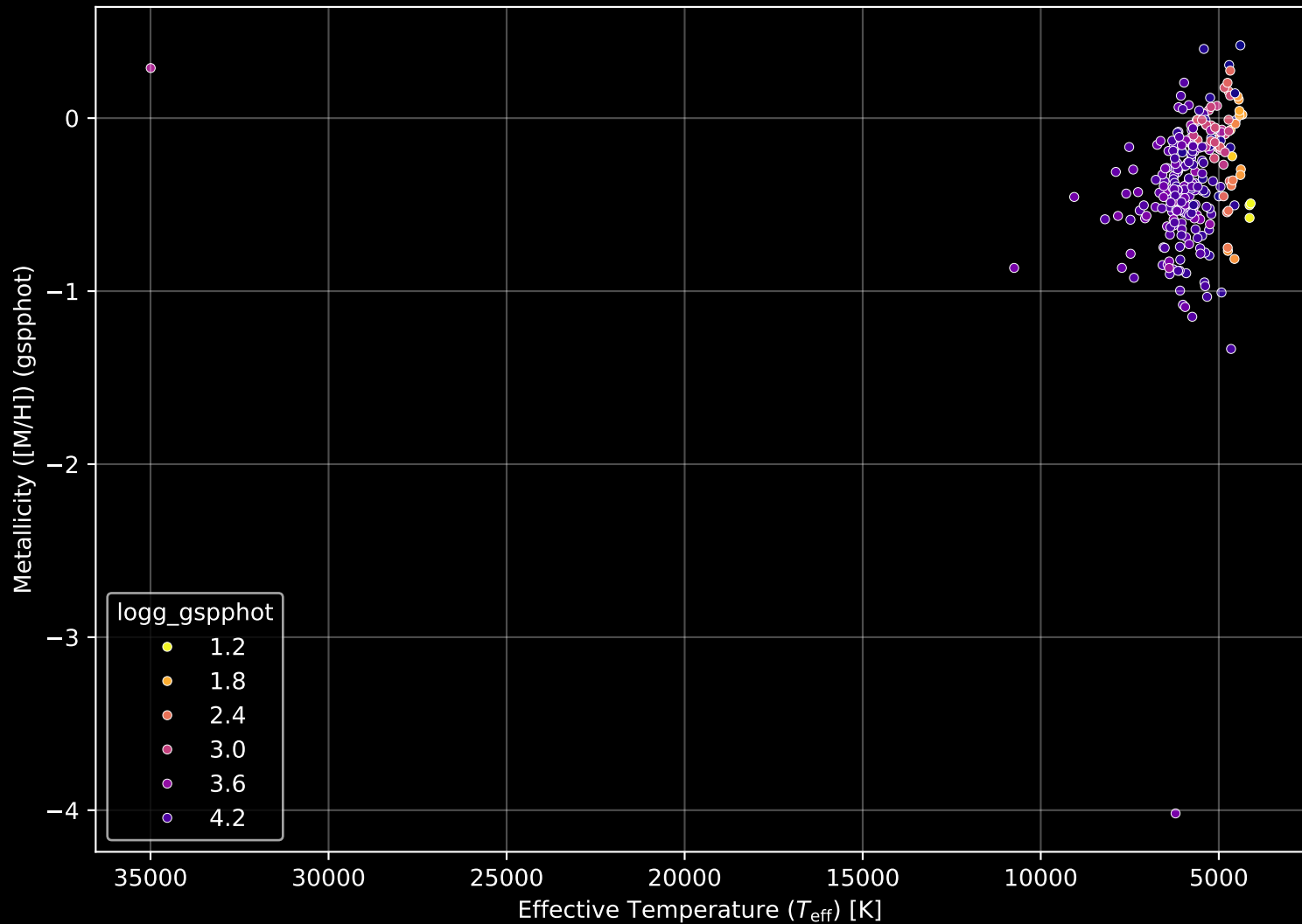
GALAH DR4 Field: [3441] Stellar Population Parameters (n= 269)
